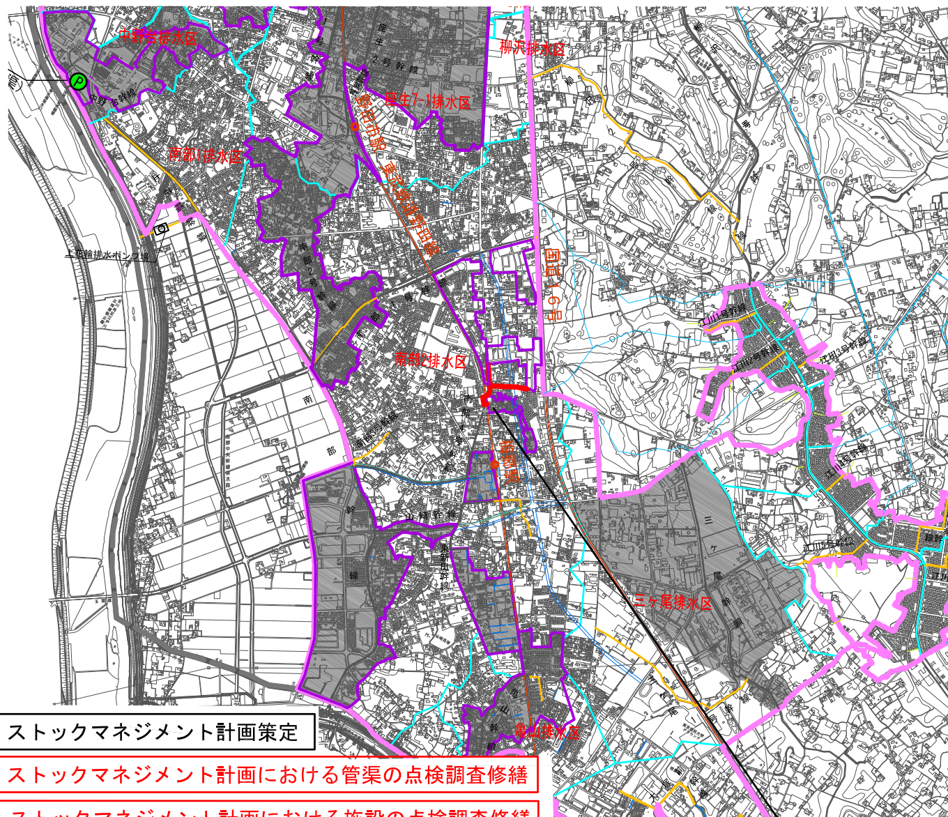
南部2排水区計画図
