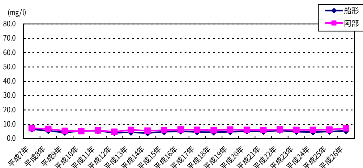
図 6-60 水質汚濁状況経年変化 （浮遊物質：SS） （利根川水域、阿部水域：関宿落堀）
