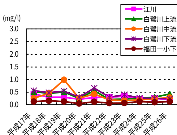
図 6-74 水質汚濁状況経年変化（全リン） （利根運河水系、江川水域）
