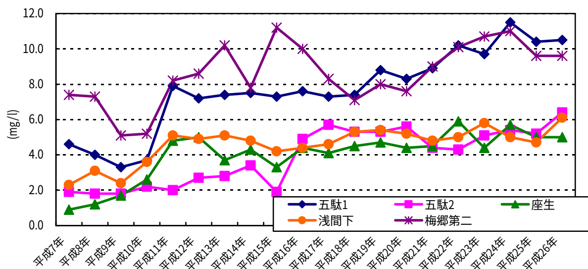
図 6-33 水質汚濁状況経年変化（溶存酸素:D0）（江戸川水系）
