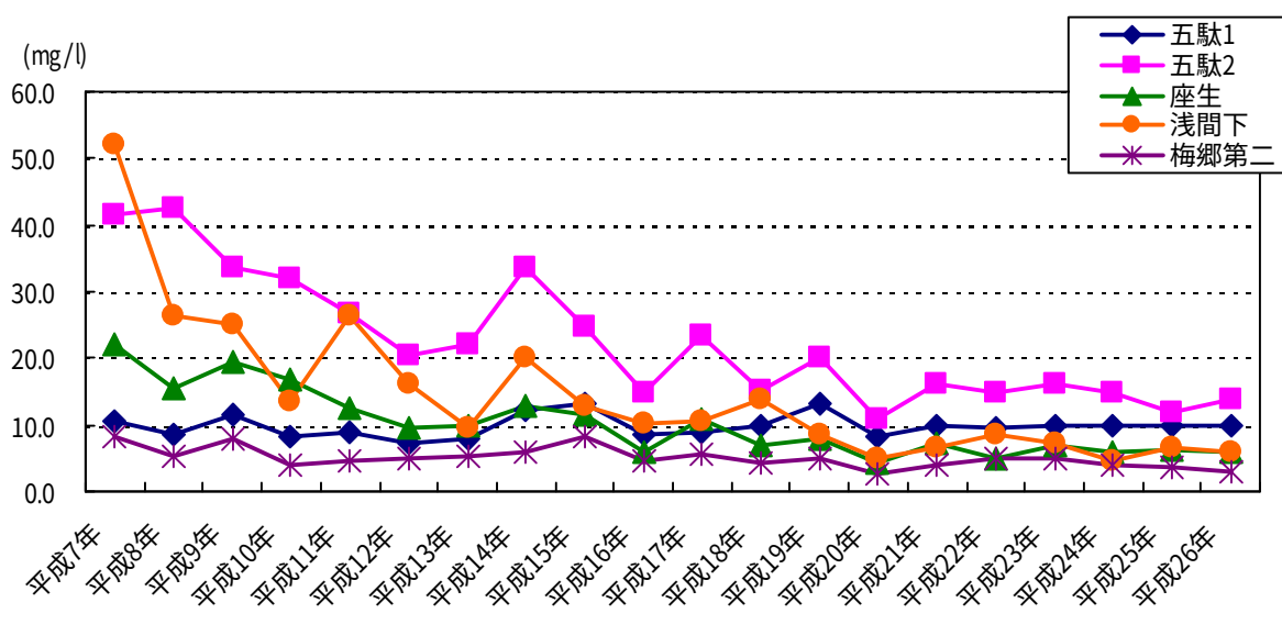
図 6-15 BOD 指標による水質汚濁状況経年変化（江戸川水系）
