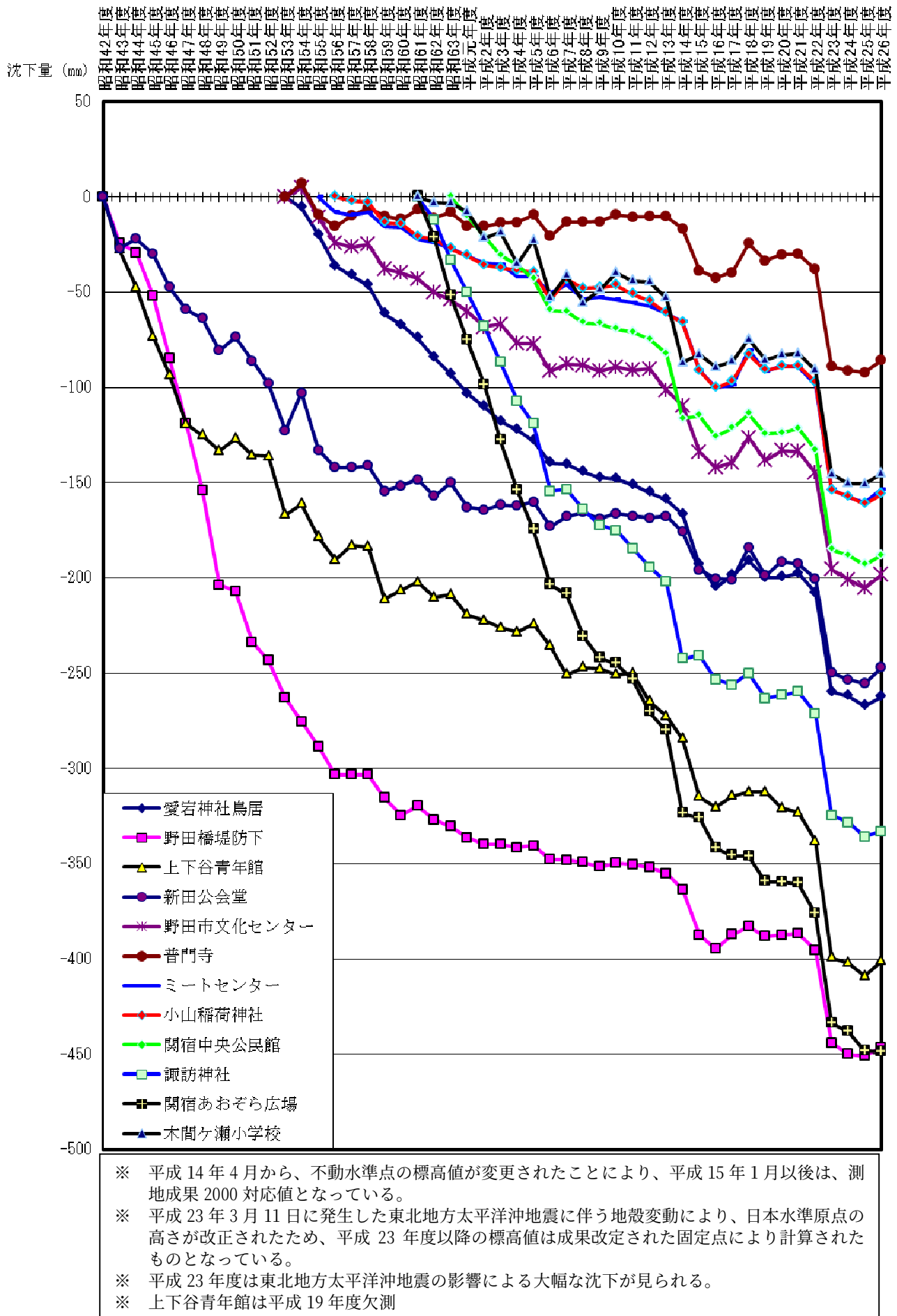
図 9-2 代表的な観測地点の経年地盤変動傾向図
