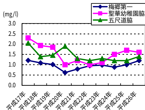
図 6-75 水質汚濁状況経年変化（全リン） （利根運河水系、その他水域）
