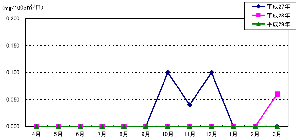
図 5-18 アルカリろ紙法による硫黄酸化物の月別測定結果（農林業センター）
