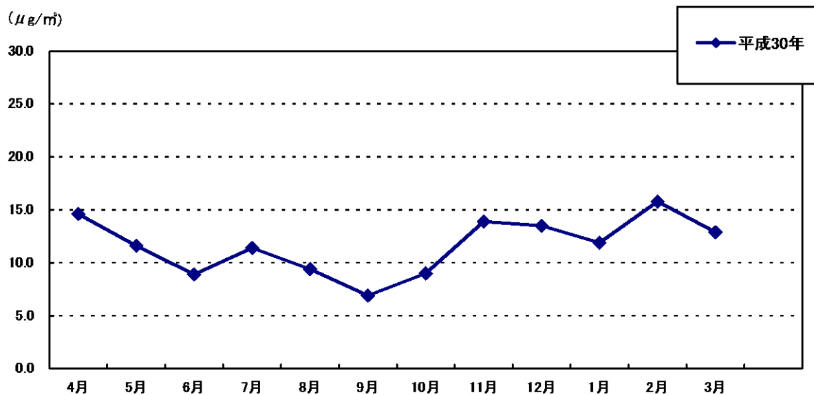
図 5-16 大気汚染桐ヶ作測定所における微小粒子状物質 (PM2.5) の月別測定結果
