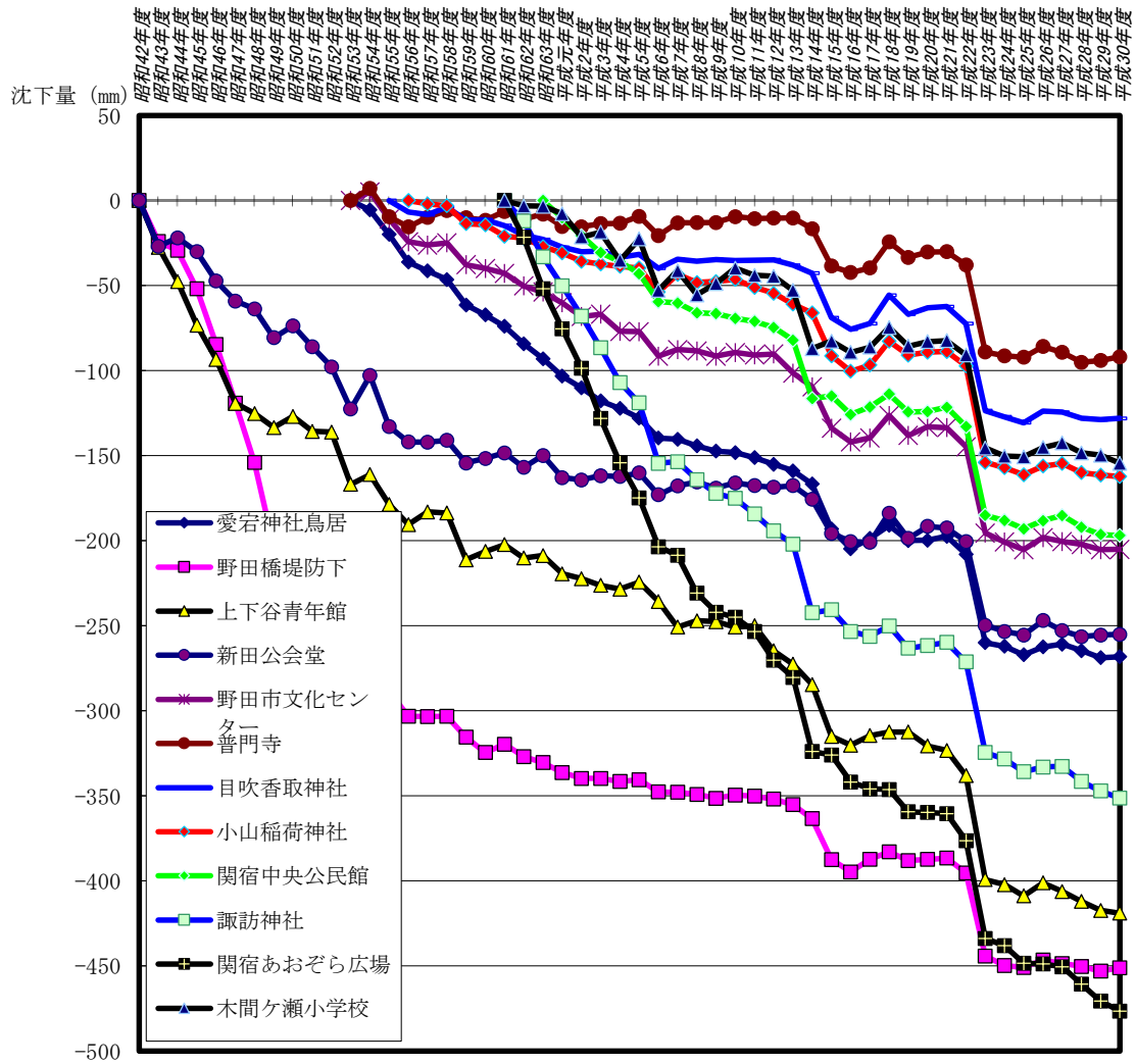
図 9-2 代表的な観測地点の経年地盤変動傾向図
