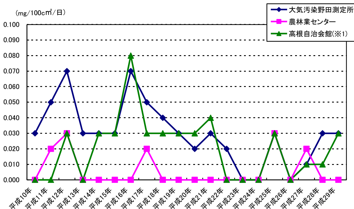
図 5-20 アルカリろ紙法 (※2) による硫黄酸化物の経年変化 (年平均値)
