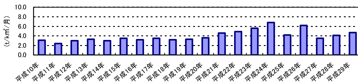
図 5-23 ダストジャー中の降下ばいじんの平均値の経年変化
