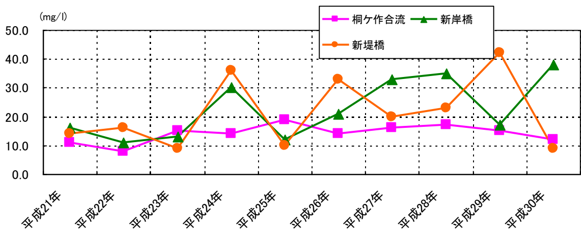
図 6-21 水質汚濁状況経年変化（浮遊物質量：SS）（利根川水域、阿部水域：関宿落堀）
