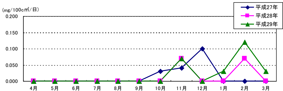
図 5-19 アルカリろ紙法による硫黄酸化物の月別測定結果（高根自治会館※1）
