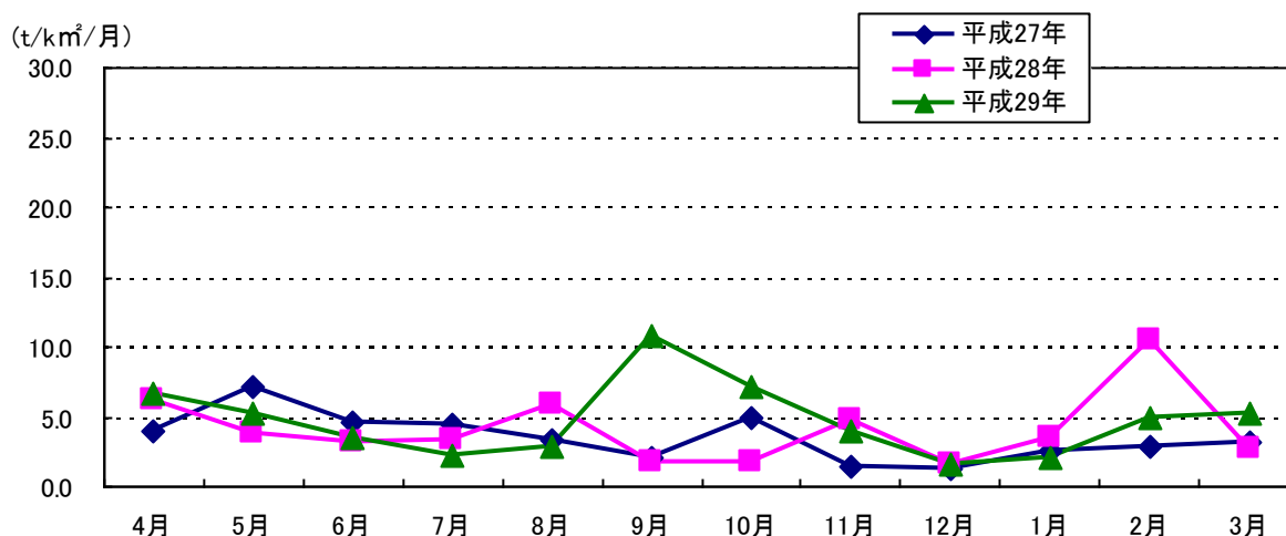
図5-21 降下ばいじんの月別測定結果（大気汚染野田測定所）
