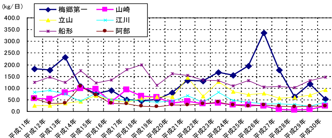
図 6-15 BOD 指標による水質汚濁負荷量経年変化（利根運河・利根川系）
