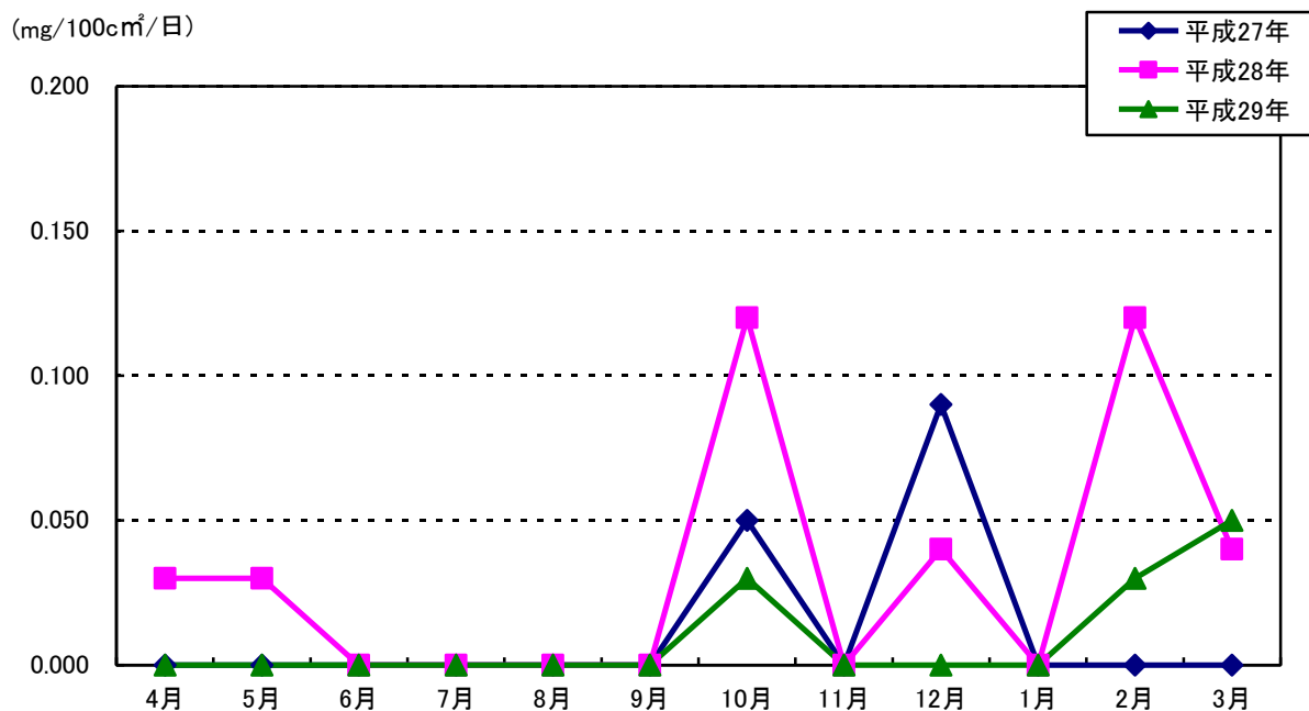
図 5-17 アルカリろ紙法による硫黄酸化物の月別測定結果（大気汚染野田測定所）
