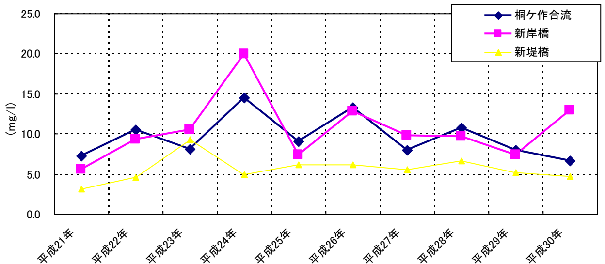
図 6-20 水質汚濁状況経年変化（溶存酸素：DO）（利根川水系）
