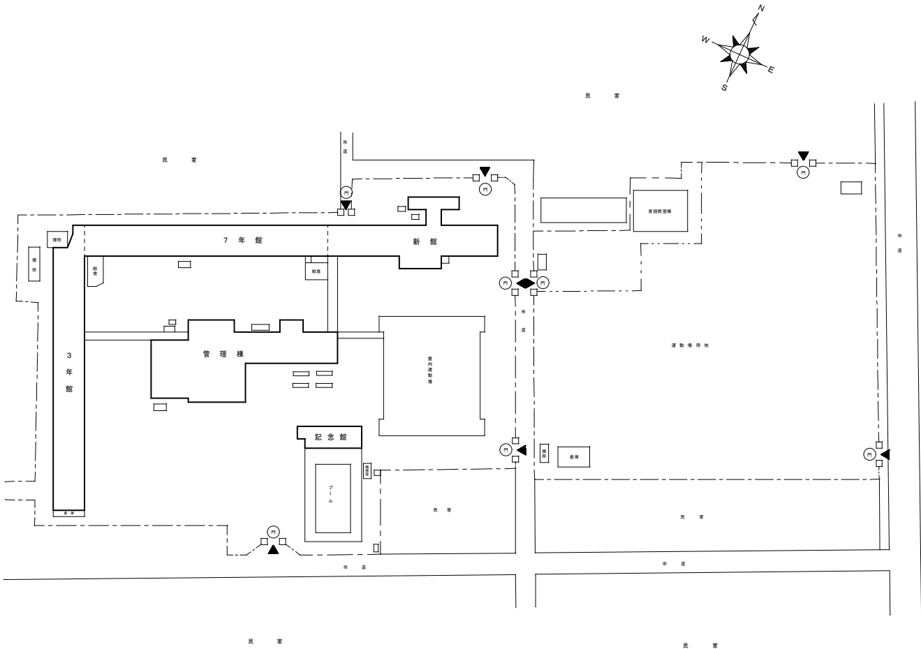
配置図
