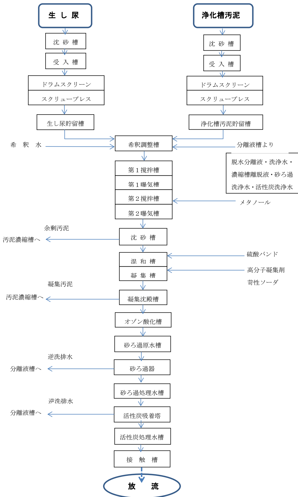
図 4-2-1 処理工程図（水処理）
