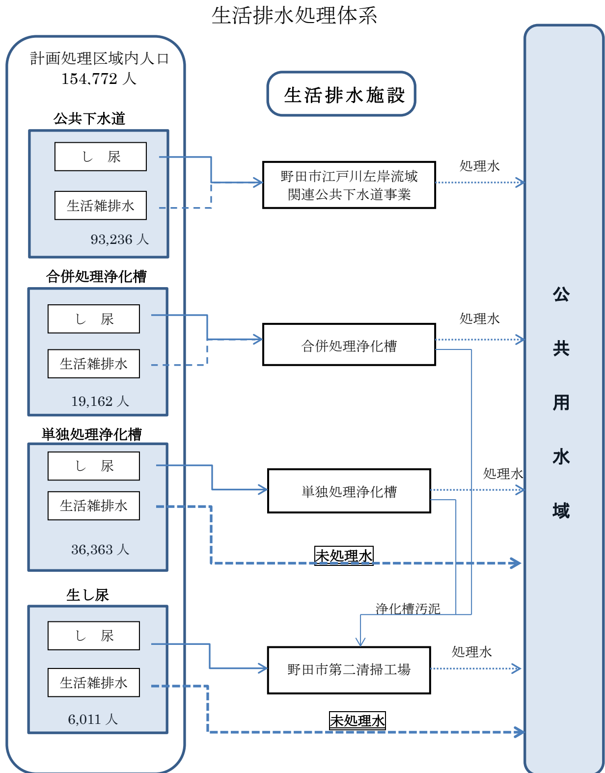
図3-1-1 生活排水処理体系
