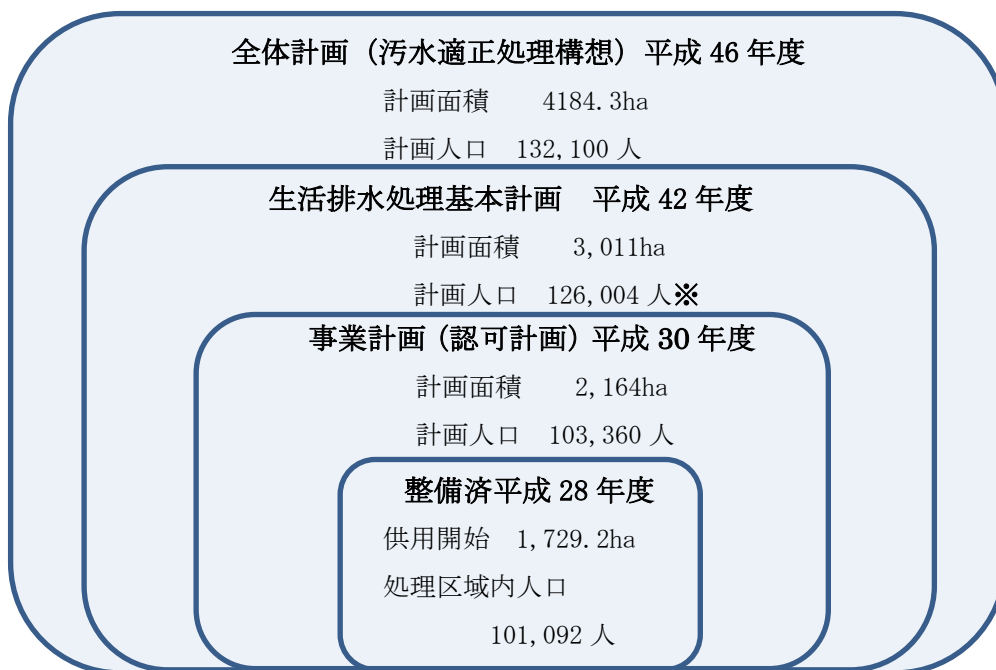
図6-1-1 下水道計画の概念図
