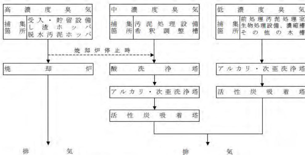
図 4-2-3 処理工程図(臭気処理)
