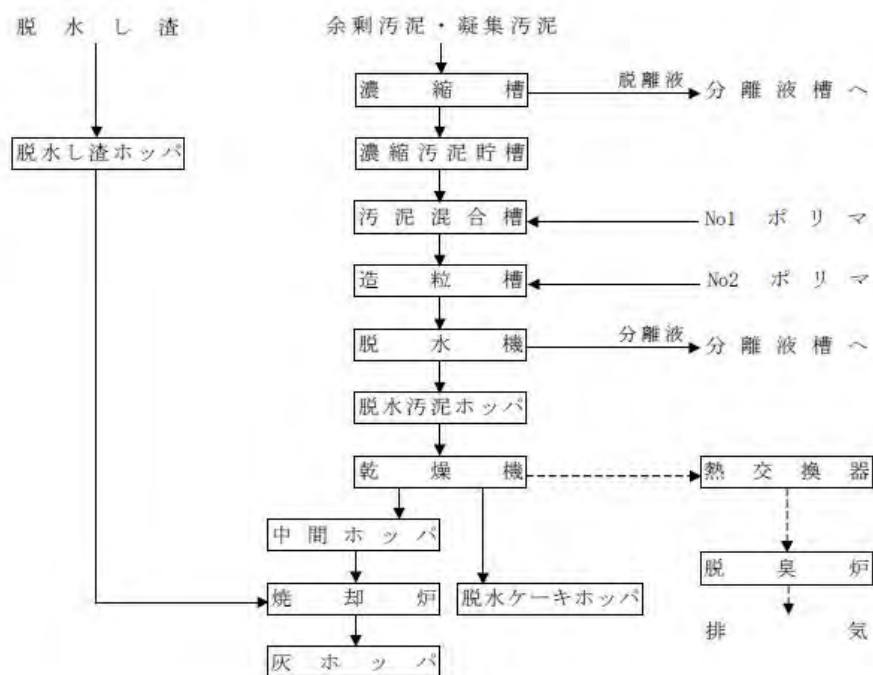
図 4-2-2 処理工程図(汚泥処理)
