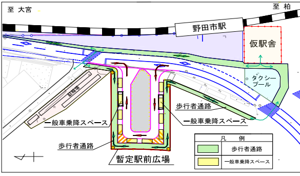
■野田市駅暫定駅前広場
