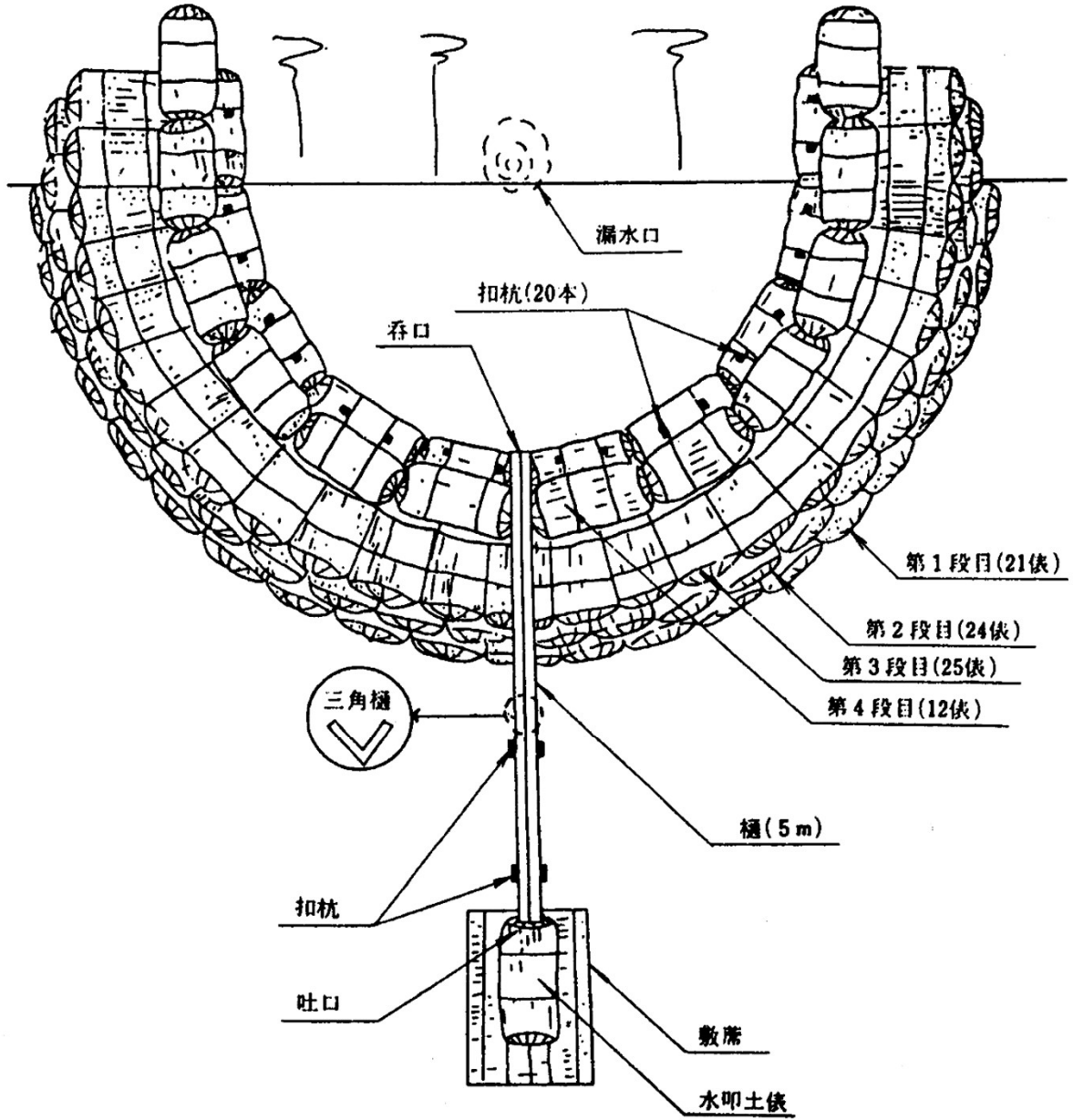
平面图 (完成)
