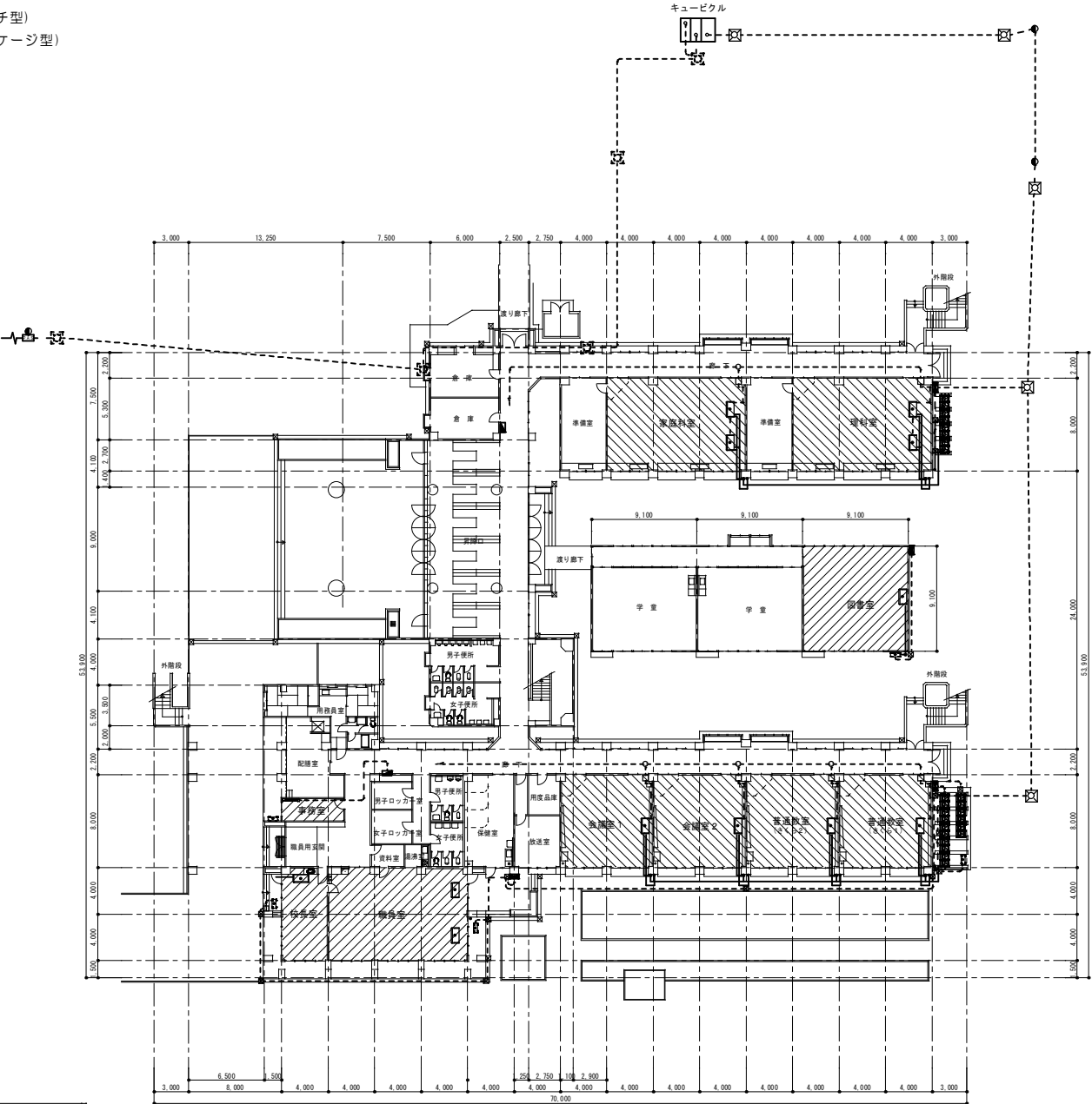
1 階平面図
