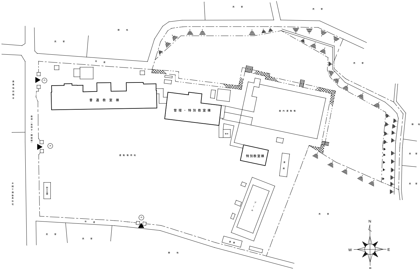
配置図
