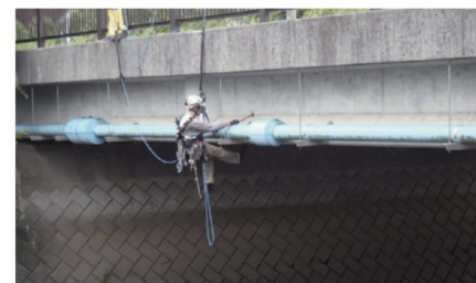
ロープで安全を確保しながら作業員が水道管を直接点検
