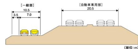
■一般部事業中間区 標準断面図（中川並行区間）
