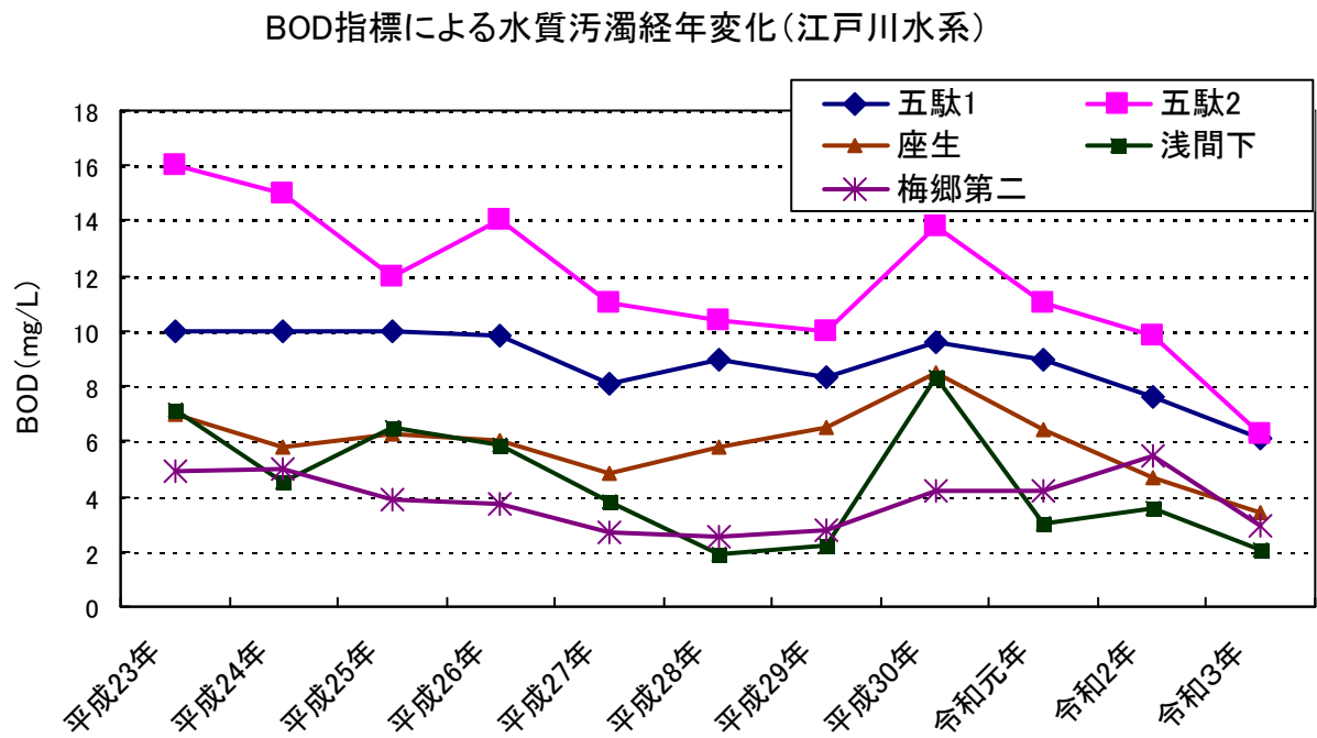
図 6-12 BOD 経年変化（江戸川水系）
