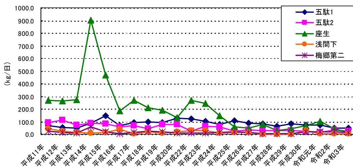
6-15 BOD 指標による水質汚濁負荷量経年変化（利根運河・利根川系）
