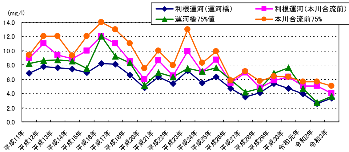
図 6-8 河川の水質汚濁状況経年変化 (DO) (利根運河)
