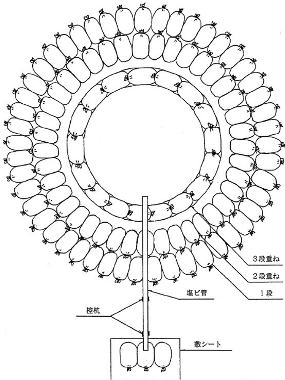
平面図 (完成) 3段
