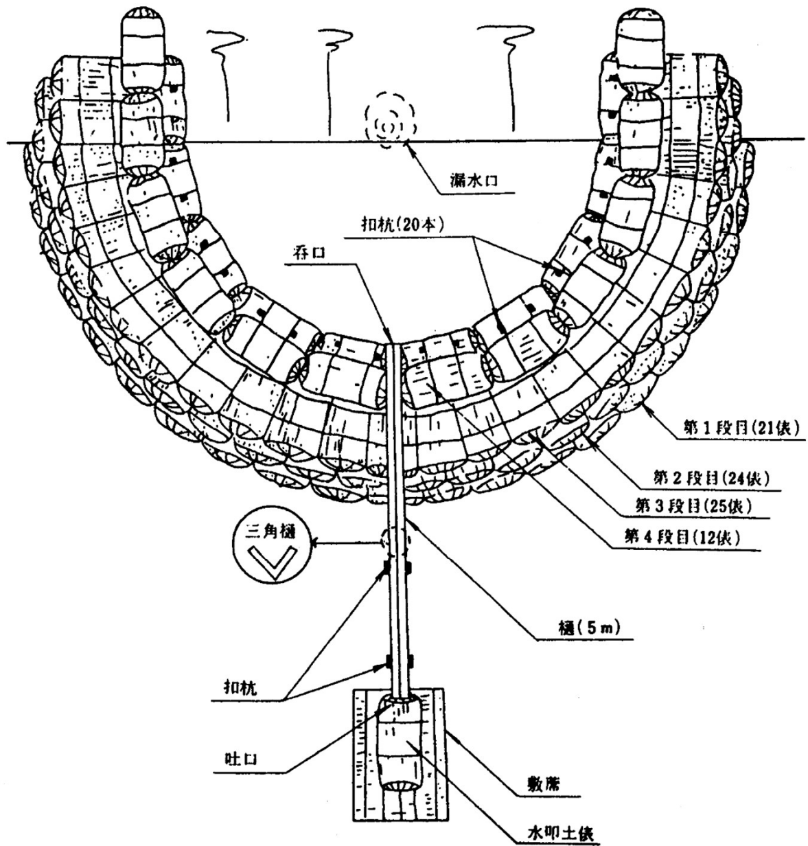
平面图 (完成)
