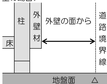
＜外壁の場合＞
